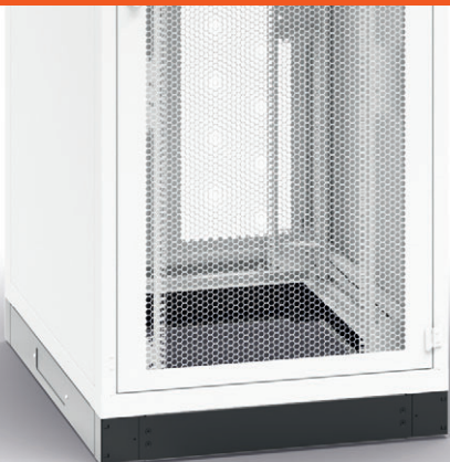
Пример модульного цоколя 800 × 1000 мм высотой 100 мм. См. рис. ниже.
